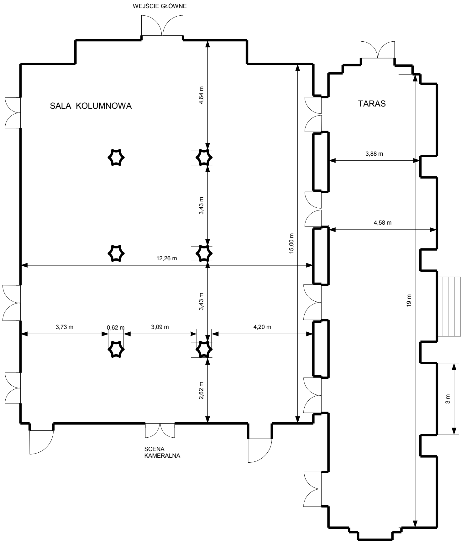
WROCŁAWSKI TEATR LALEK SALA KOLUMNOWA I TARAS RZUT POZIOMY SKALA 1:100
